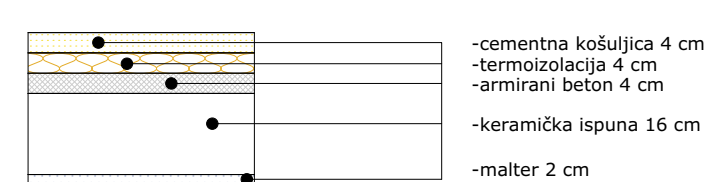
MKS- MEĐUSPRATNA KONSTRUKCIJA
