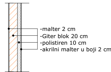
SFZ - SPOLJNI ZID (34cm)
