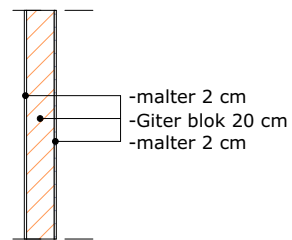
UZ1 - PREGRADNI ZID (24cm)
