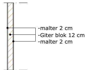
UZ3 - PREGRADNI ZID (16cm)
